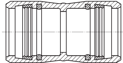
Beispiele für elastomergedichtete Verbindungen
